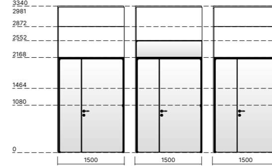
RH/LH DOUBLE HINGED DOORS PORTE DOPPIE BATTENTI DX/SX
